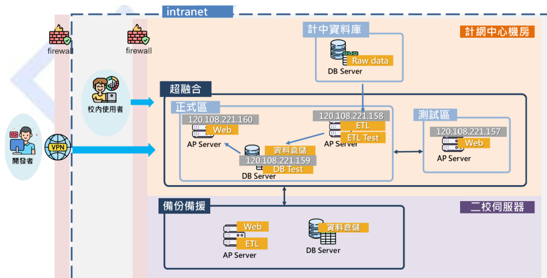
圖 5-1-1 校務大數據資料庫系統之主機環境架構圖
